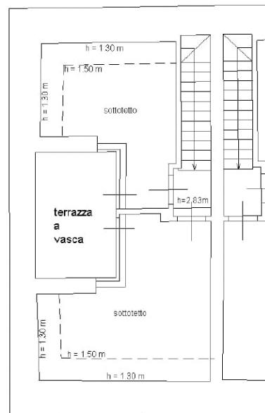
PIANTA PIANO TERZO (SOTTOTETTO)
